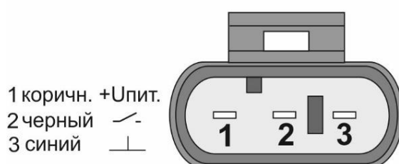
Нормально-разомкнутый контакт
