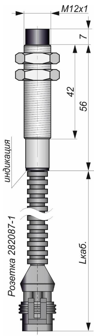
Габаритный чертеж
